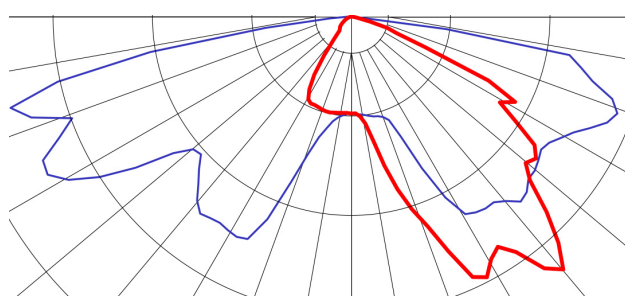
Distribuição da luz - Tipo III
