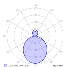
Versão Direto Indireto Opalina
