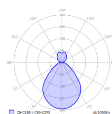
Versão direto indireto micro prismático
